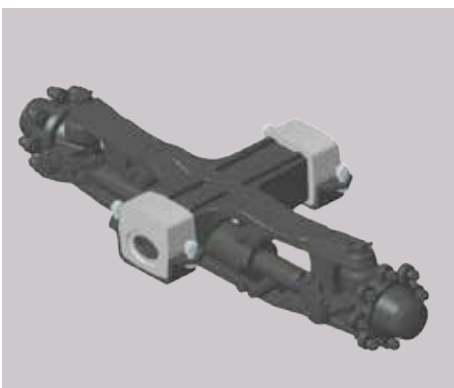
Eixo de direção fundido de serviço pesado • Carcaça do eixo reforçada • Articulação de direção com rolamento cilíndrico: maior resistência a impactos • Amortecimento em borracha: menos vibração
